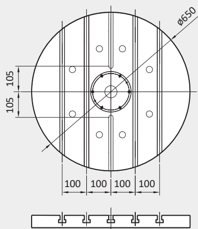
STÓŁ UCHYLNIO-OBROTOWY
