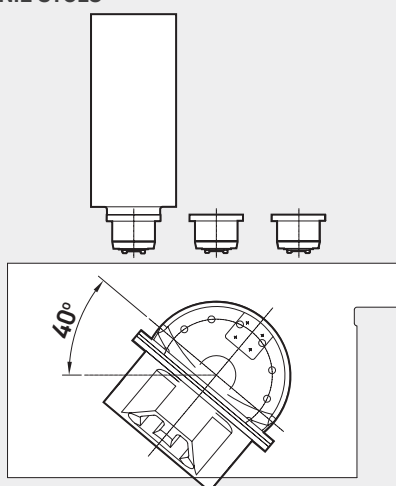
PRZECYCHYLENIE STOŁU
