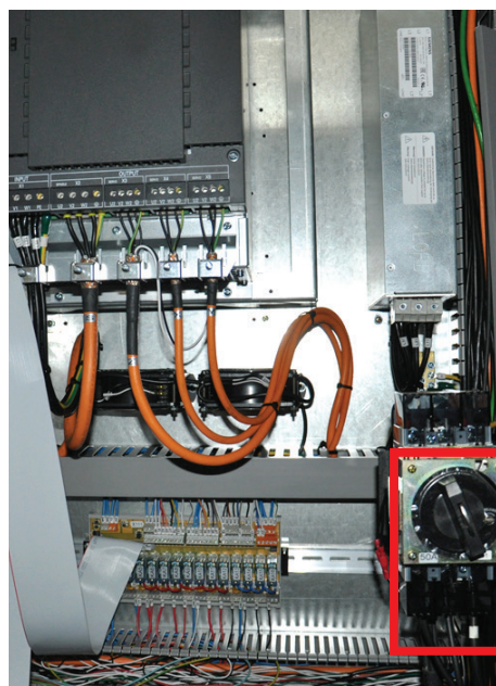
ZASILANIE ELEKTRYCZNE
